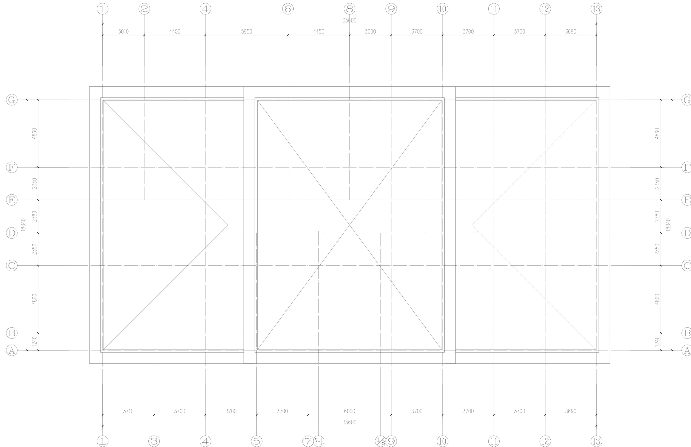
屋顶层平面图:100
