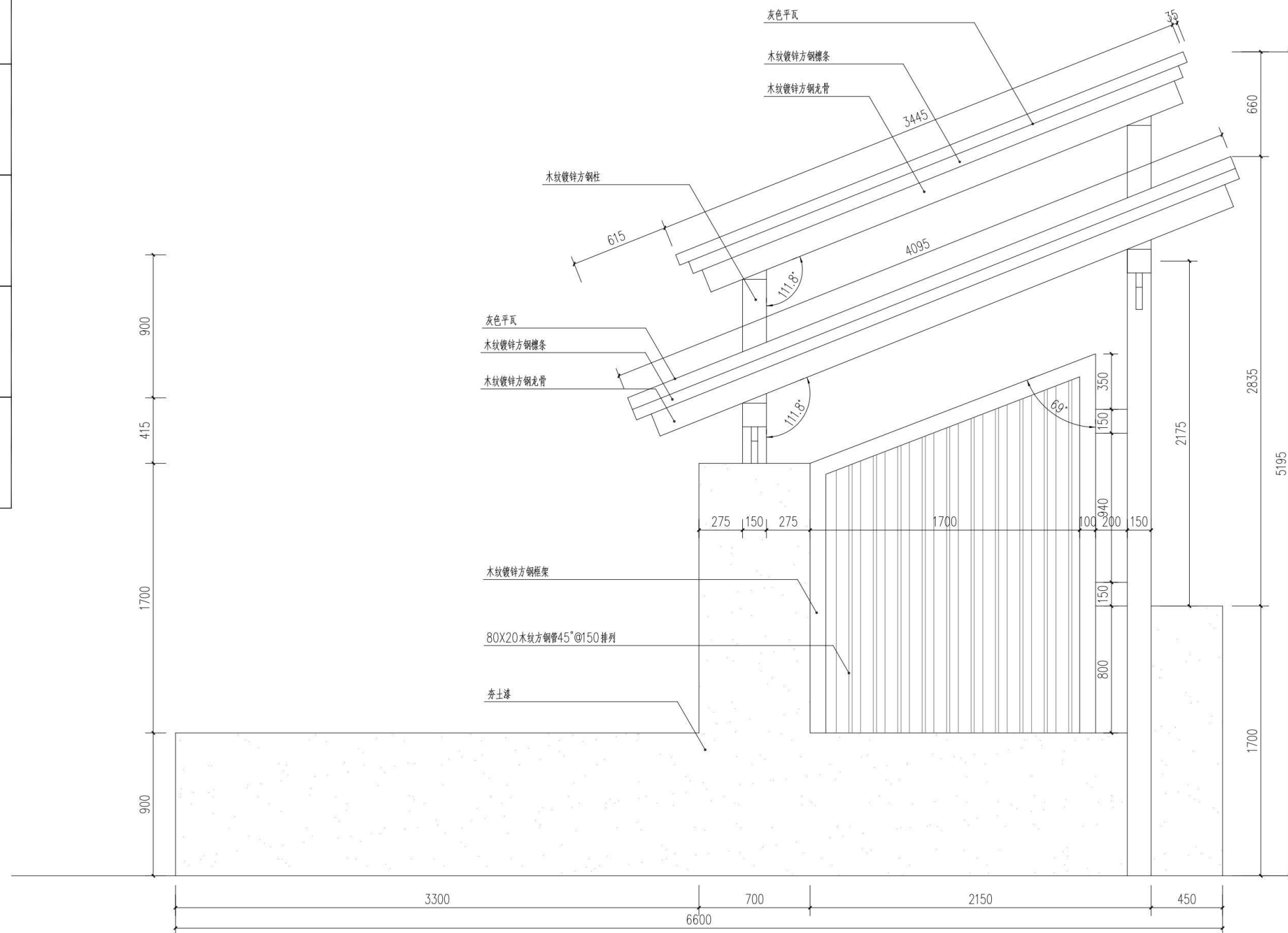
①景观构架立面图 1:20
