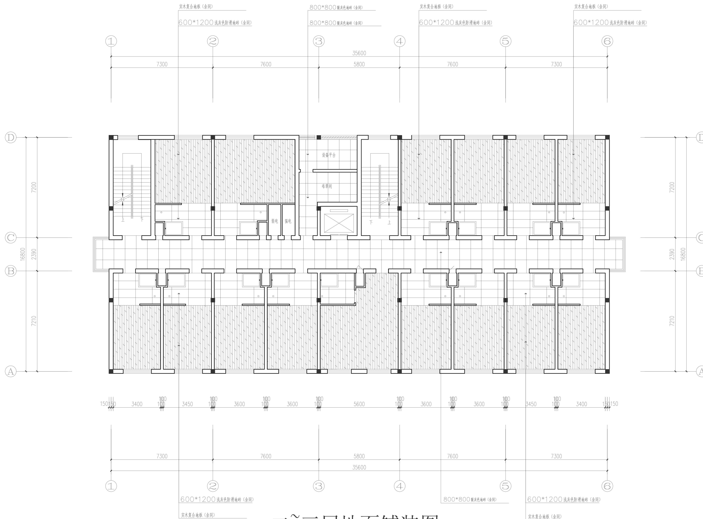
二~三层地面铺装图
