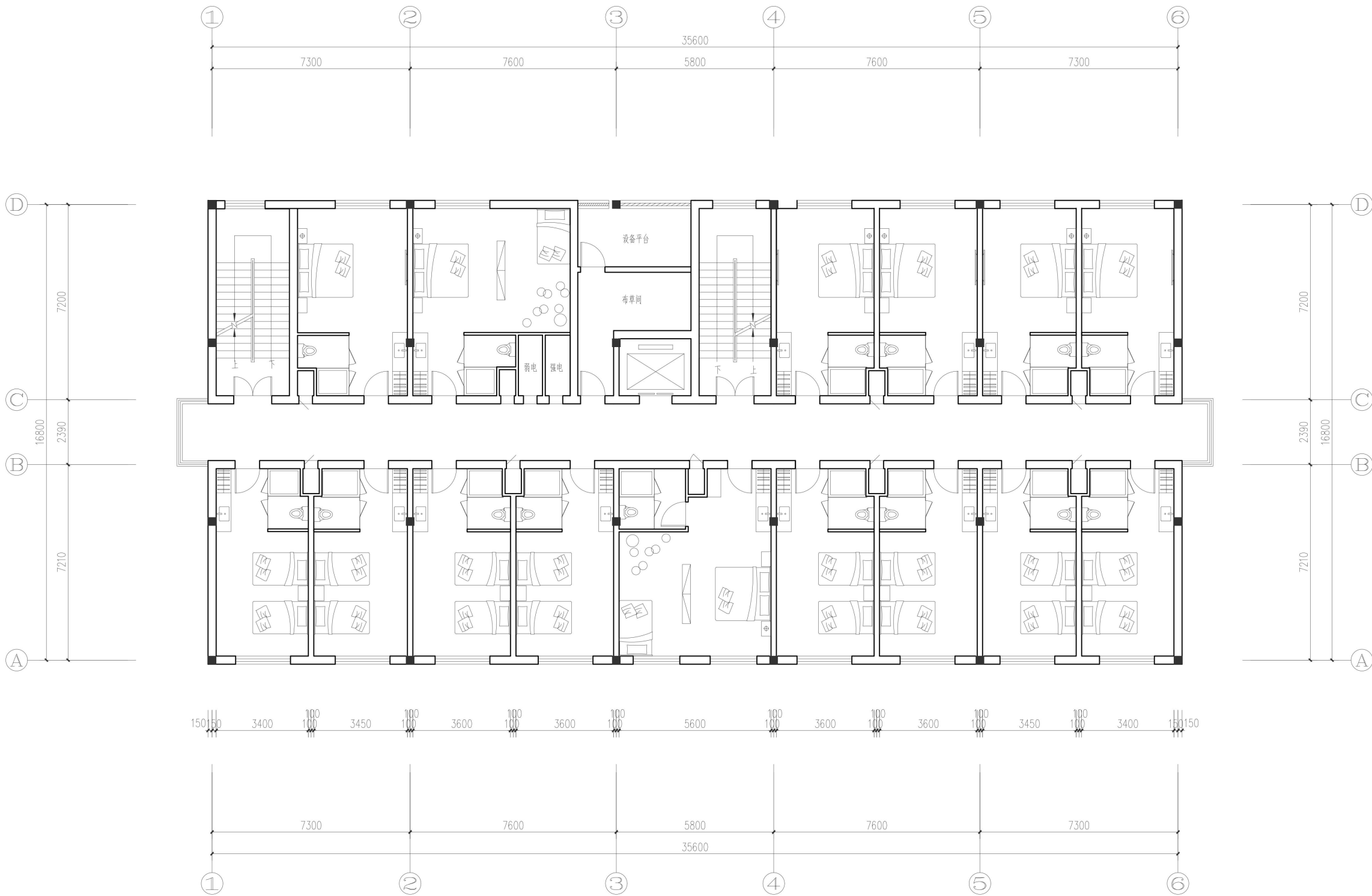
二~三层平面图
