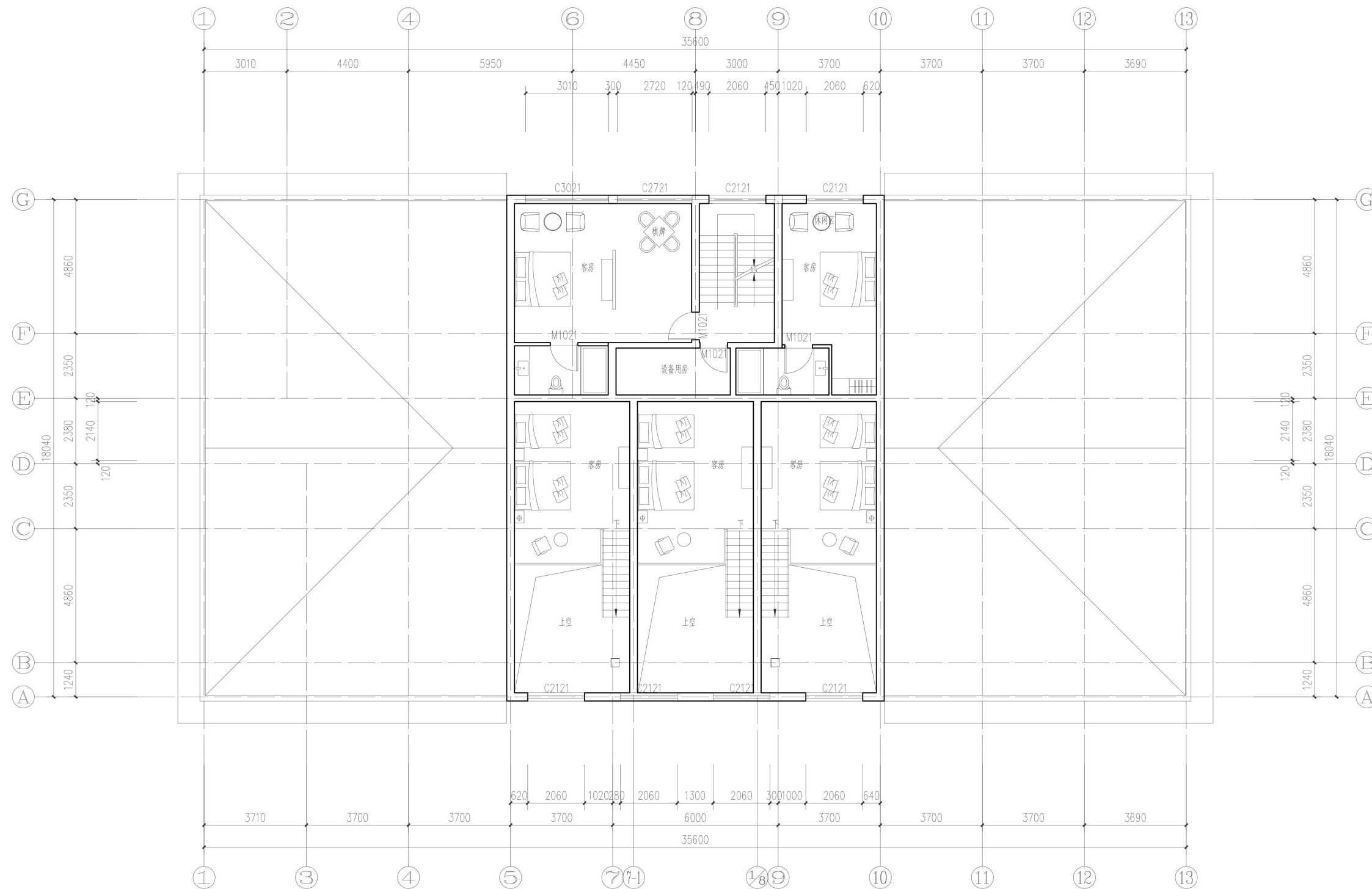
五层平面图 1:100
