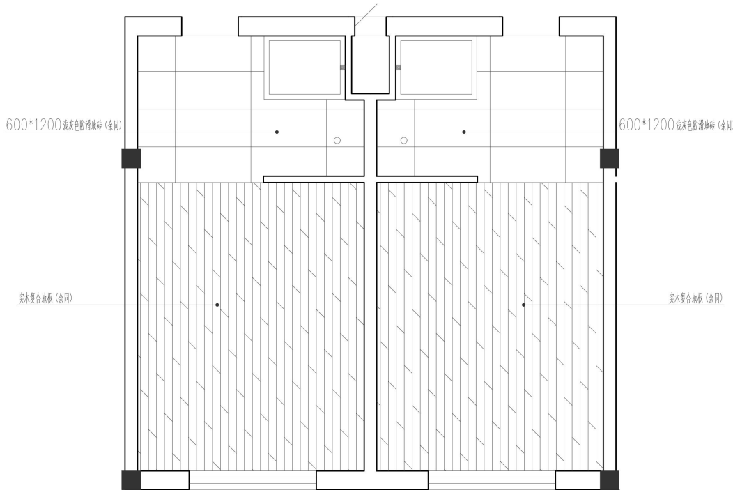
1#楼二人标间地面铺装大样图 1:50
