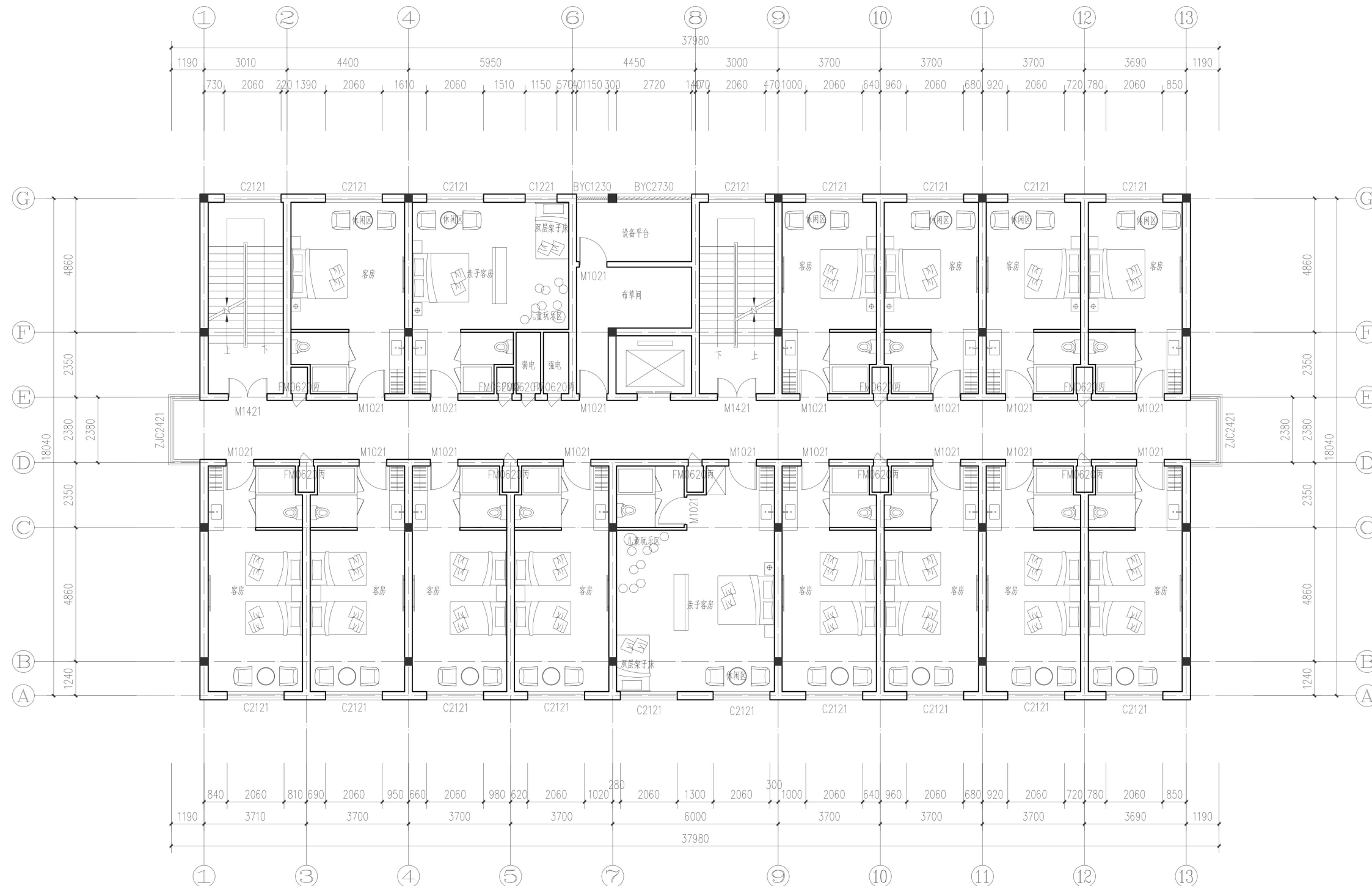
二-三层平面图 1:100
