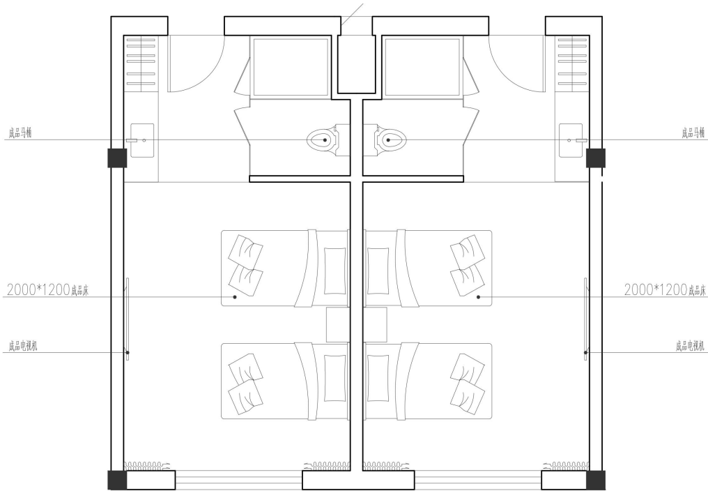
1#楼二人标间平面布置大样图 1:50
