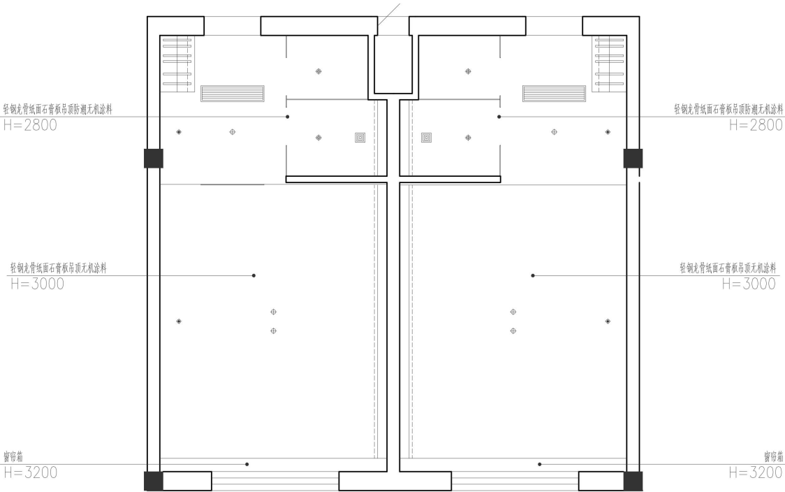
1#楼二人标间顶面布置大样图 1:50
