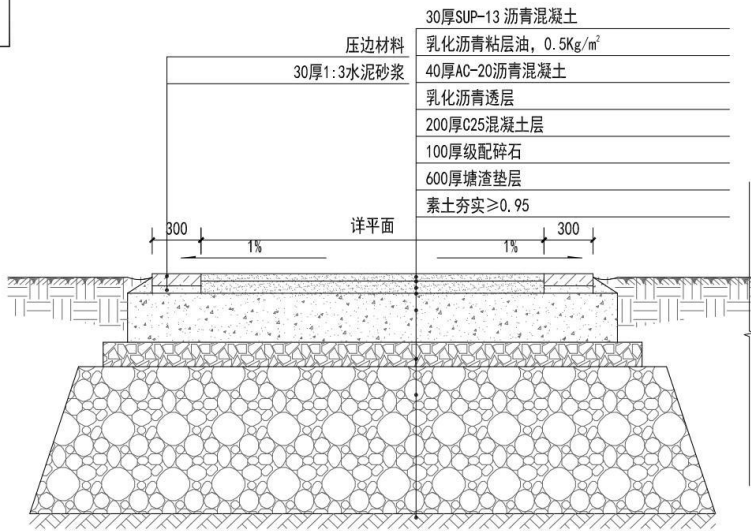
③沥青道路标准段剖面图 1:20
