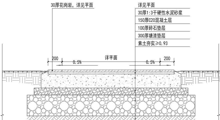
①人行道路标准段剖面图 1:20
