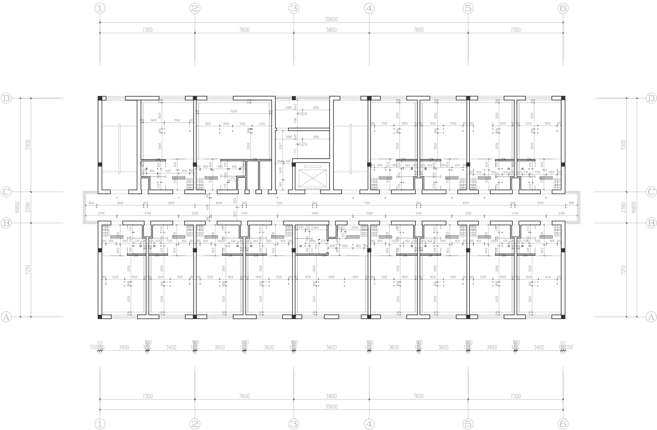
二~三层顶面灯位尺寸图
