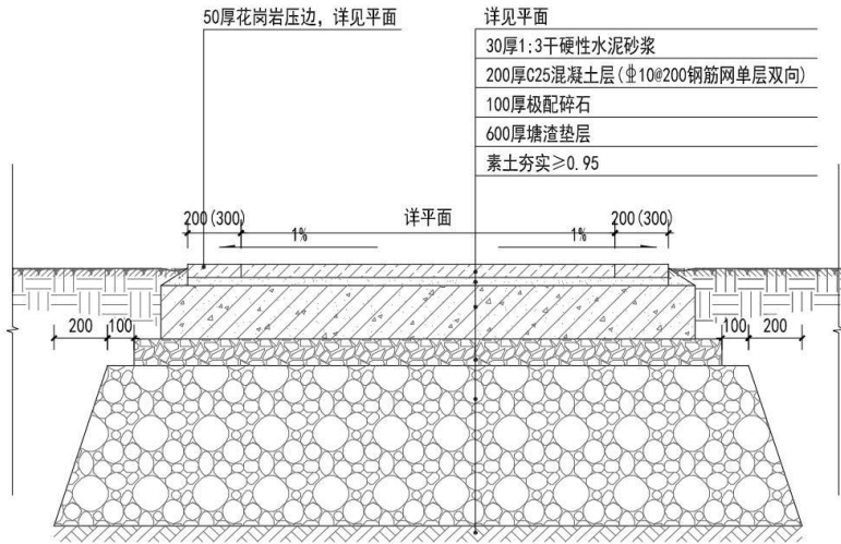
②通车道路标准段剖面图 1:20
