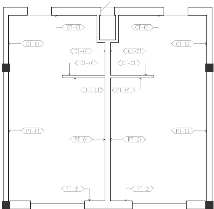
1#楼二人标间墙面完成材料图 1:50
