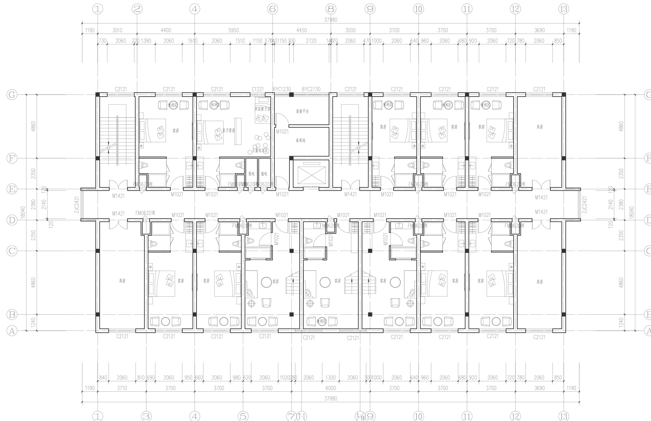
四层平面图 1:100
