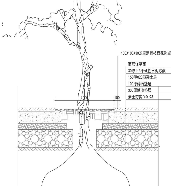
④树池通用剖面图 1:20
