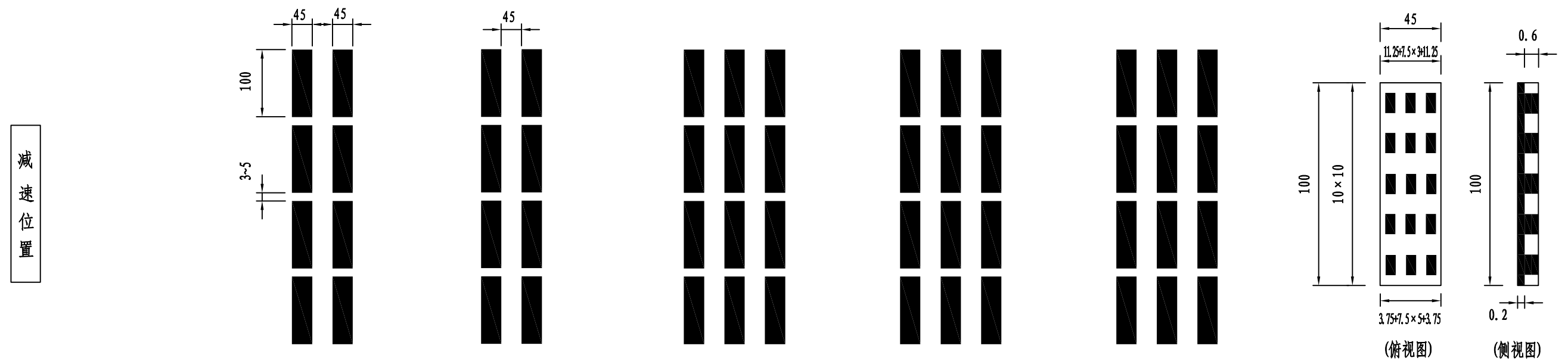
減速標線大樣圖 單條
