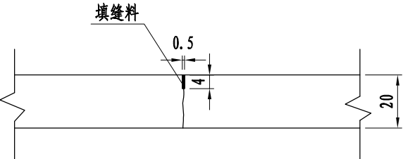
横向缩缝
