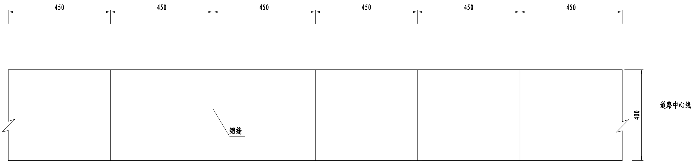
水泥板块设计图(二)
