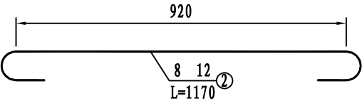
基础主筋大样图
