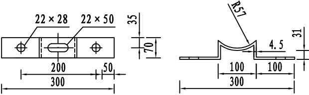
托架 (300 × 70 × 4.5)
