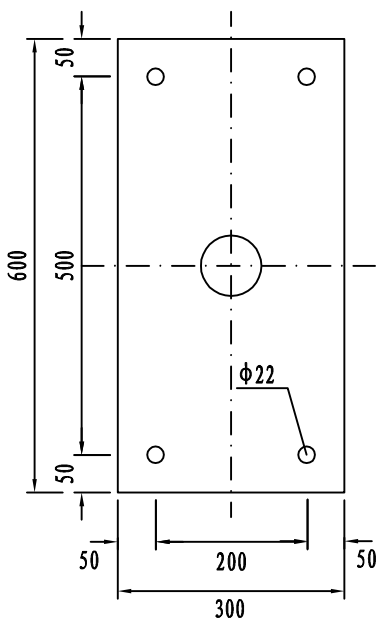
加劲法兰盘 1: 10
