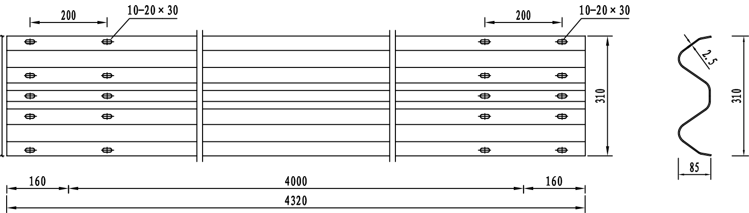
波形梁护栏板 (310 × 85 × 2.5)
