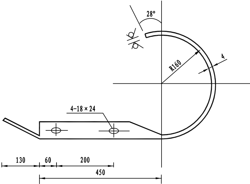
平面图 1:8
