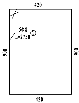
基础箍筋大样图 1: 20
