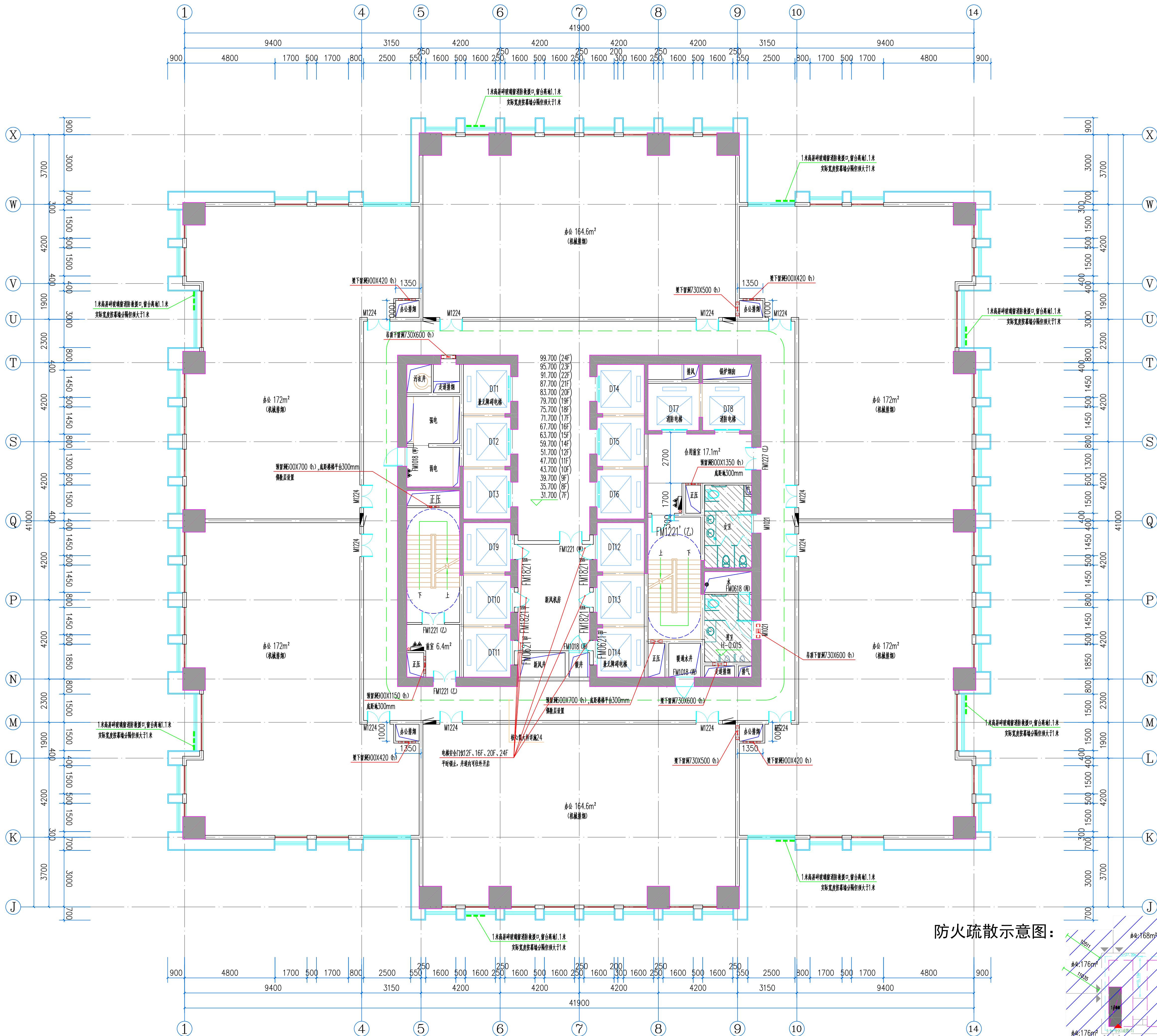
七~十二、十四~二十四层（办公）平面图 1:100
