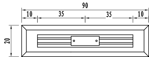
标志板背面连接图
